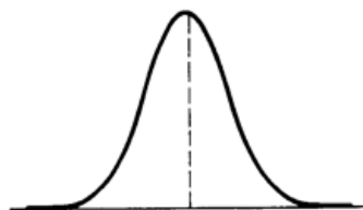
Figuur 1. Normale verdeling.
