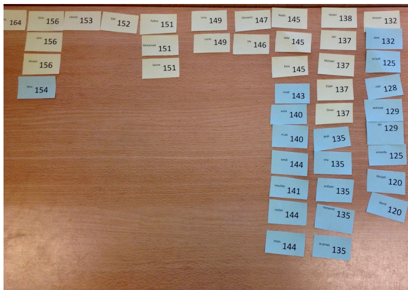
Afbeelding 3. In categorieën vergeleken.
