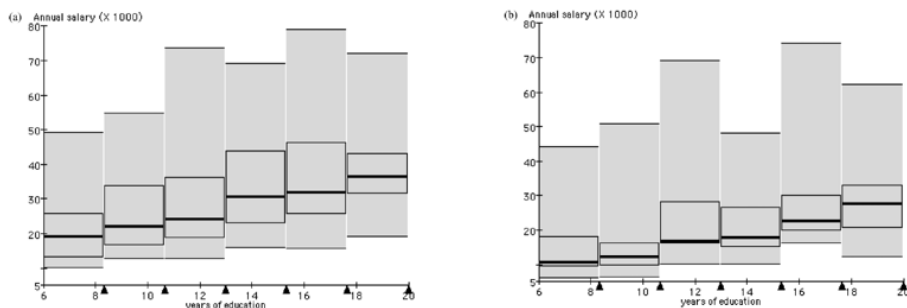
Figuur 16 a en b. Salarisontwikkeling van leraren. (Gefingeerde data.)
