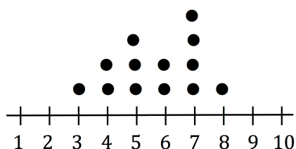
Figuur 17. Gangbare vorm van een dot plot.
