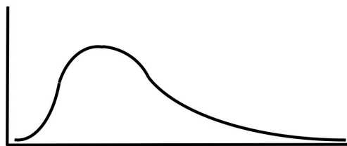
Figuur 2. Scheve verdeling.
