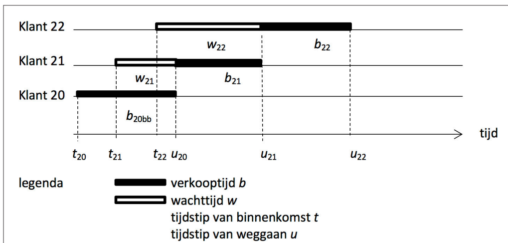
Grafiek 1. Grafische weergave van het verloop van een wachtrij. Toelichting:
