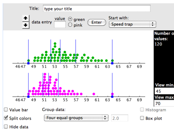
Figuur 18. Snelheidsdata ingedeeld in vier gelijke groepen.
